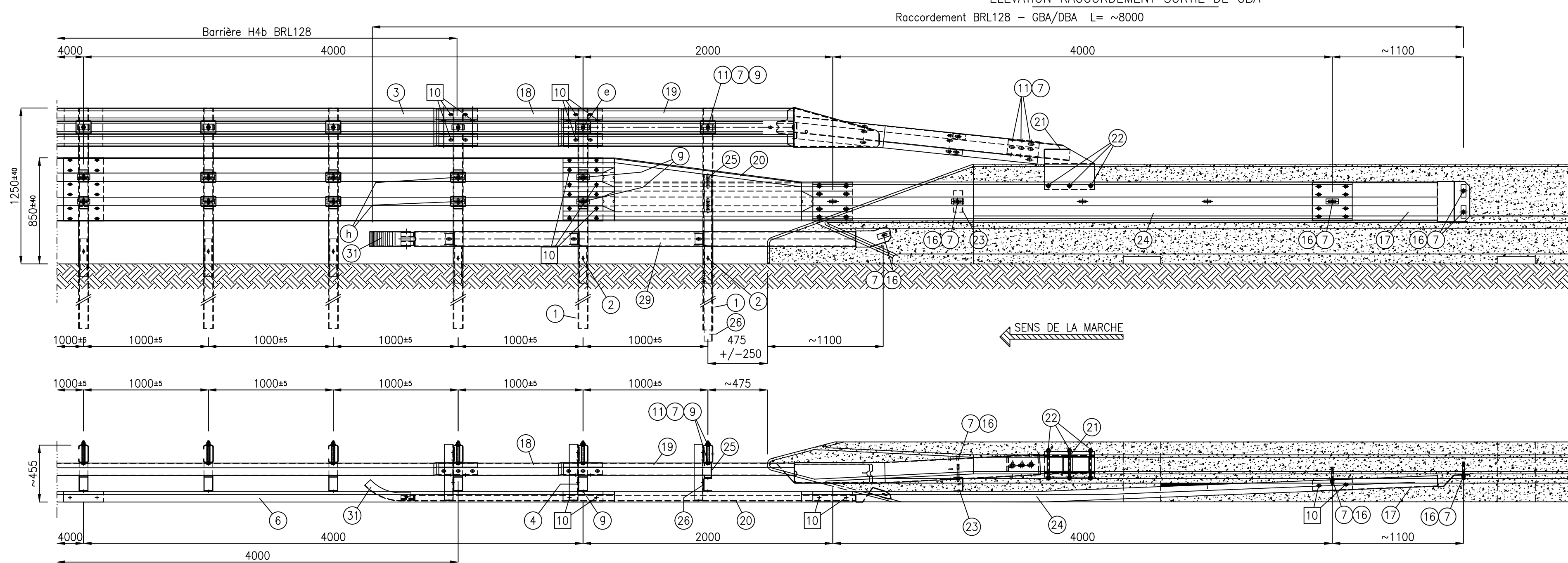
ELEVATION RACCORDEMENT SORTIE DE GBA
