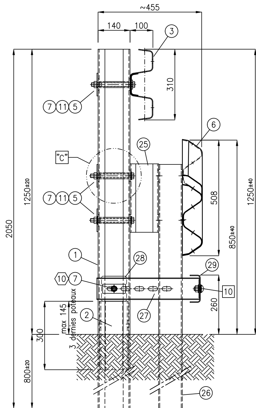
COUPE B-B ECHELLE 1:10
