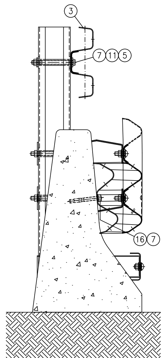
COUPE A-A ECHELLE 1:10
